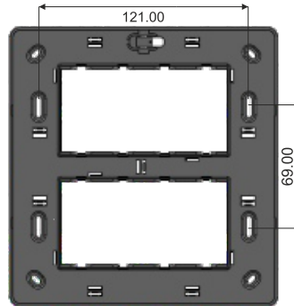
8 Module (Square) 154 x 161 *
