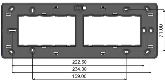
8 Module (Horizontal) 263 x 93 *
